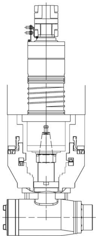
756 自動交換 90 度銑頭
